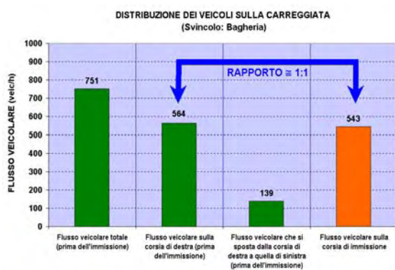
Figura 11 – Distribuzione delle portate veicolari (Svincolo di Bagheria).
